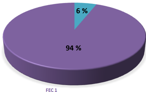
FEC sans D4Z4
